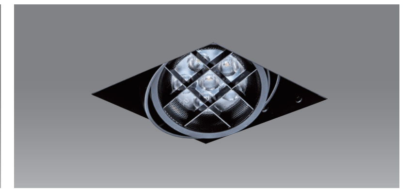
嵌入孔 161x161 mm CT-90654 (嵌入式) 適用光源 LED A~H 材質 鋁框鋼材 顏色 White Black (訂製品) 功能 可調角度 尺寸 L160mm W160mm H155mm
