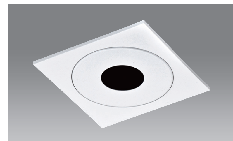
CT-91273 光源 MR16 LED A~F 材質 鋁製品 顏色 □ White 功能 可調角度 尺寸 L89mm W89mm H60mm
